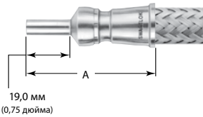
Тип облицовочного сварного шва — 1/4 и 1/2 дюйма
