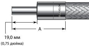
Тип ручного сварного шва — все прочие размеры
